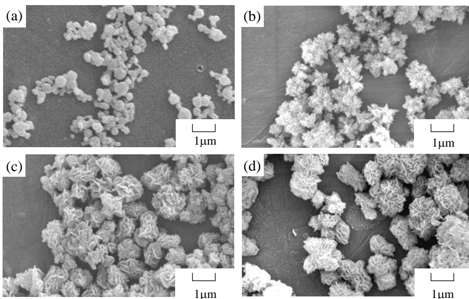
図2 解像度が高い良好な写真の例。目的物質の繊細な表面構造が存分に表現されている。遠山岳史氏（日本大学）にご提供頂いた。
